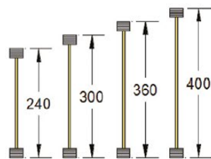
52x35 mm LVL Flange 9.5 mm OSB Web
