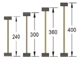
90x38 mm LVL Flange 11 mm OSB Web
